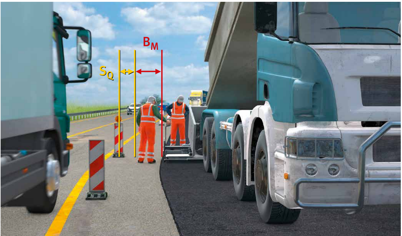
Abb. 100 Erforderlicher Arbeitsraum ( B_M ) und Sicherheitsabstand ( S_Q )
