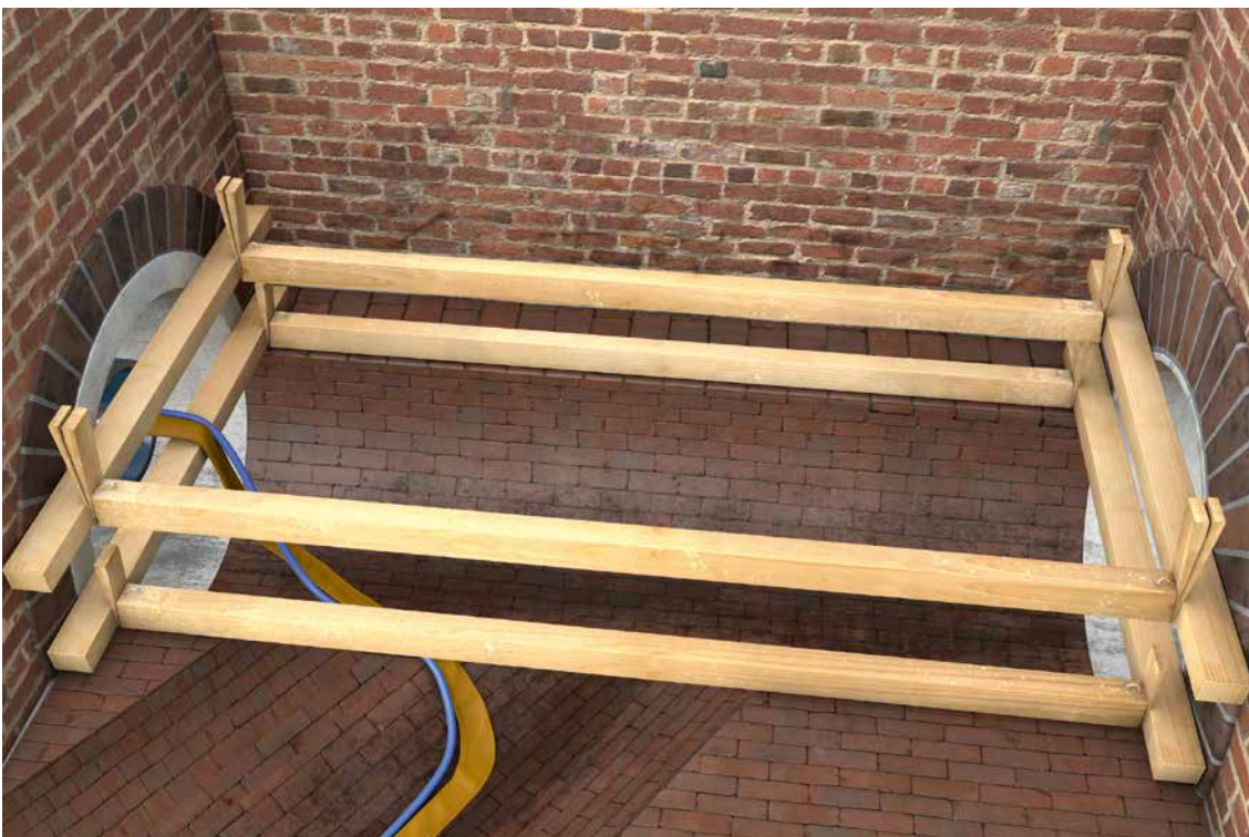
Abb. 118 Formschlüssige Ausschubsicherung mittels zimmermannsmäßigem Verbau
