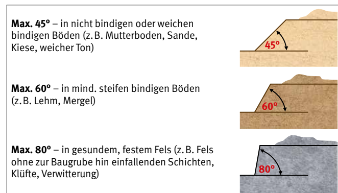
Abb. 105 Zulässige Böschungswinkel – bis zu einer Tiefe von 1,25 m können bei standfestem Boden senkrechte Grabenwände hergestellt werden
