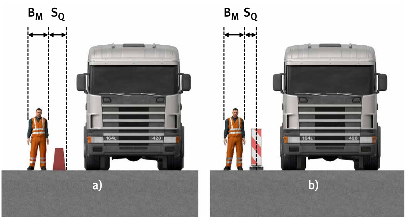
Abb. 11 Bezugslinie für seitliche Sicherheitsabstände ( S_Q ) zum fließenden Verkehr: a) dem Verkehr zugewandte äußere Begrenzung bei Fahrzeug-Rückhaltesystemen b) Mittelachse bei Leitbaken, Leitkegeln, Leitwänden, Leitschwellen, Leitborden (ASR A5.2)
