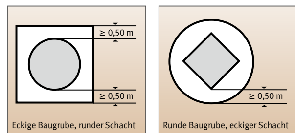
Abb. 114 Arbeitsraumbreiten für Schachtbauwerke – DIN 4124
