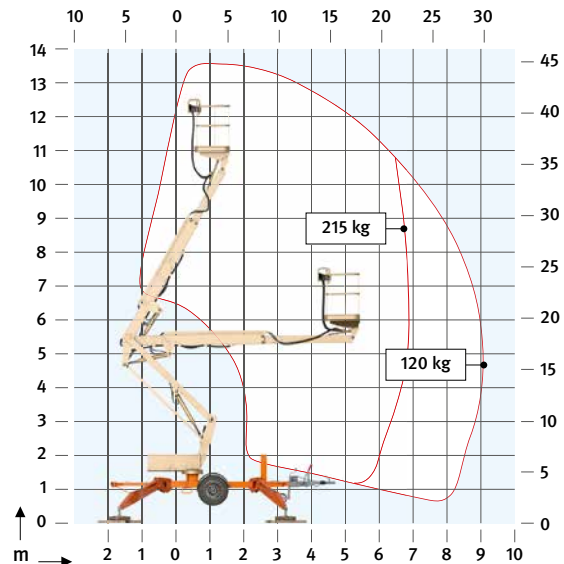
Abb. 63 Reichweitendiagramm
