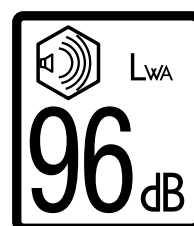
Abb. 42 Kennzeichnung des Schalleistungspegels an einer Maschine
