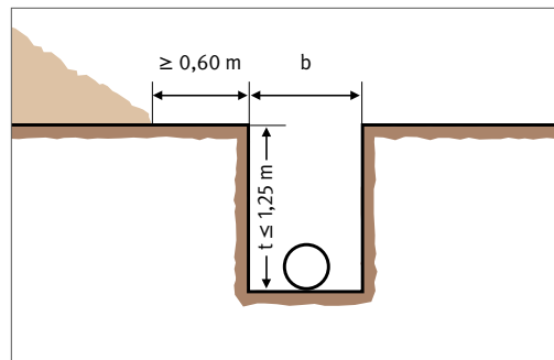
Abb. 106 Baugruben bis 1,25 m Tiefe
