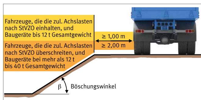
Abb. 108 Sicherheitsabstände von Fahrzeugen, Baumaschinen oder Baugeräten bei nicht verbauten Baugruben und Gräben mit Böschungen
