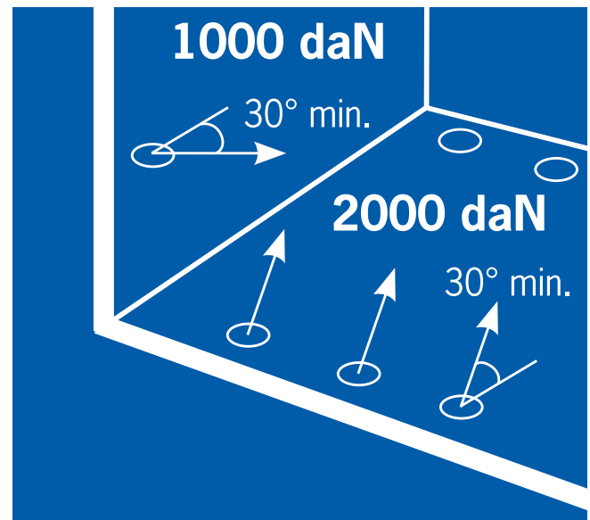
Abb. 84 Kennzeichnung von Zurrpunkten
