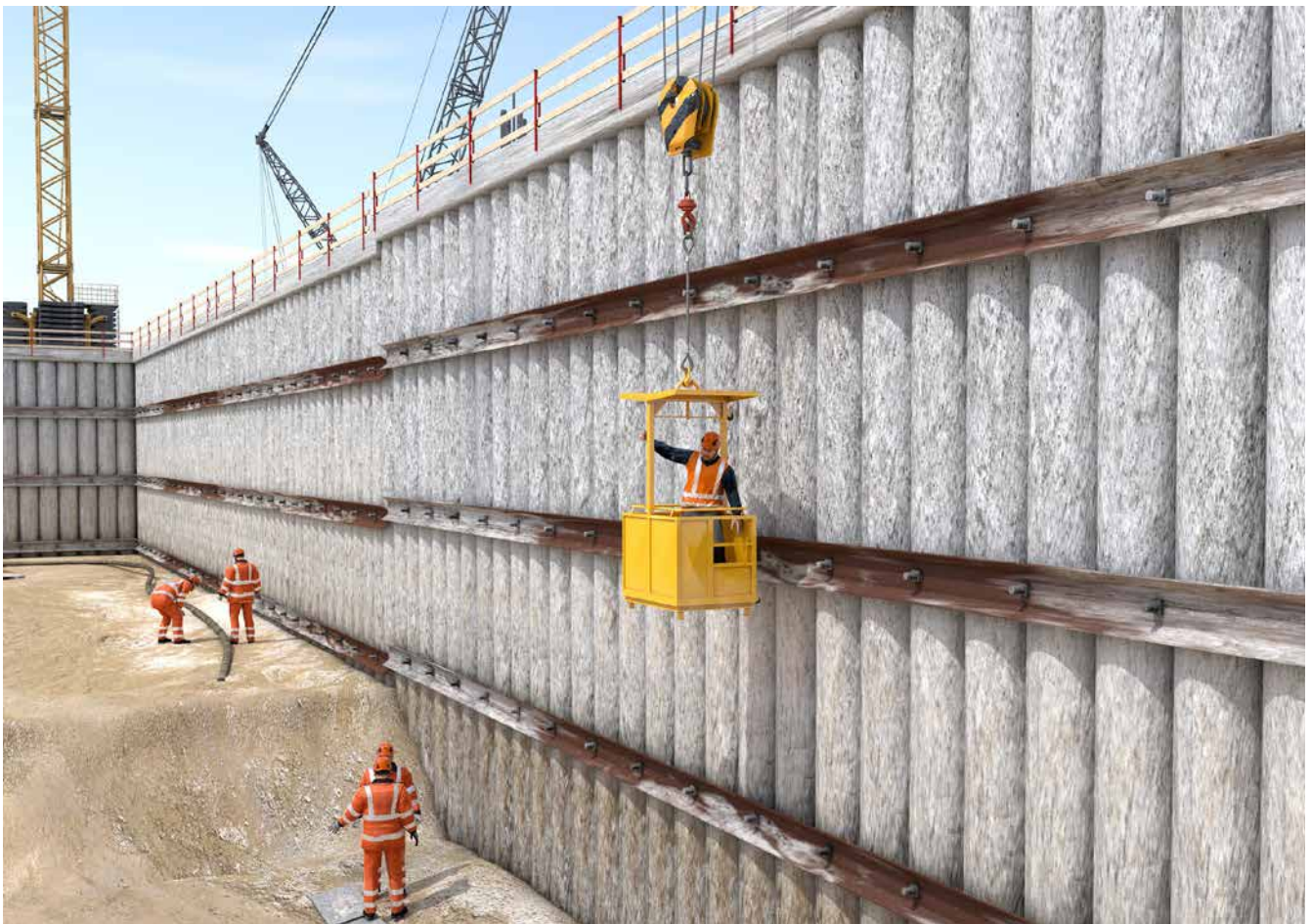
Abb. 90 Hochziehbares Personenaufnahmemittel (PAM)
