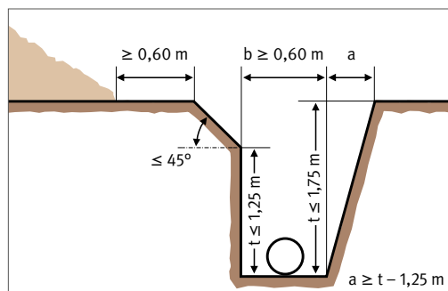
Abb. 107 Baugruben bis 1,75 m Tiefe
