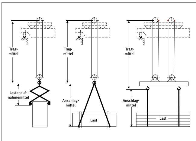
Abb. 86 Prinzipskizze Tragmittel, Lastaufnahmemittel, Anschlagmittel
