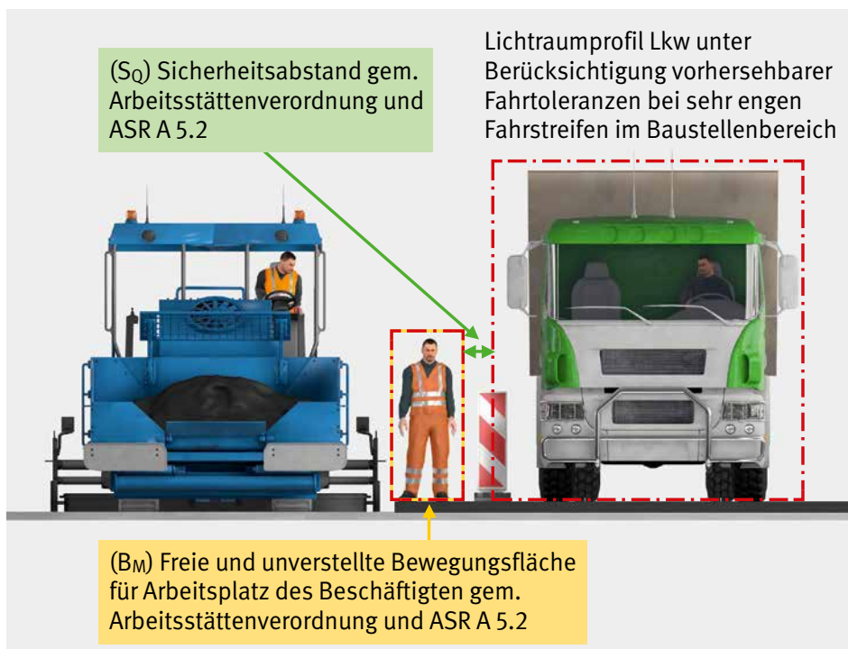
Abb. 10 Sicherheitsabstand und freie, unverstellte Bewegungsfläche nach ArbStättV
