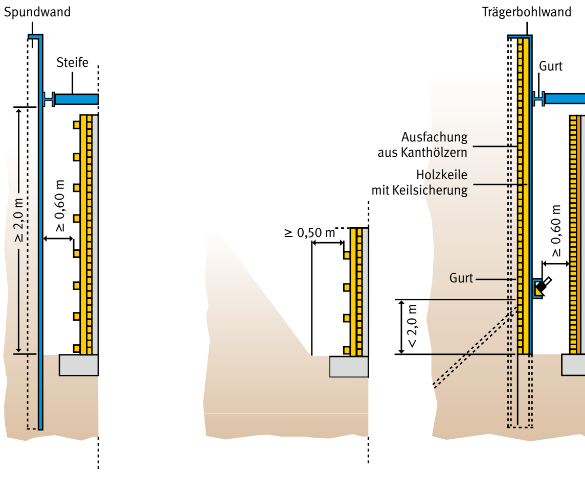
Abb. 113 Arbeitsraumbreiten nach DIN 4124
