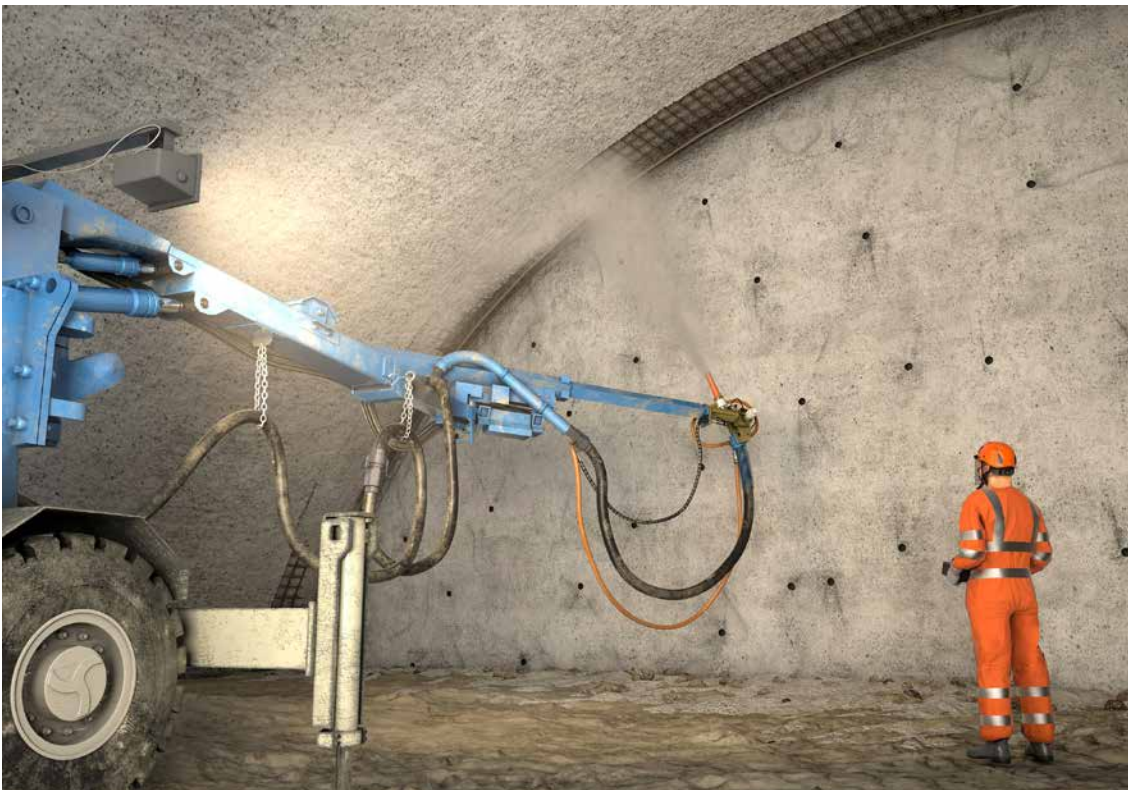
Abb. 138 Einsatz von Naßspritzbeton und Manipulator
