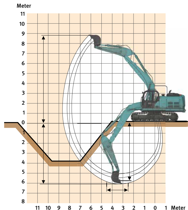
Abb. 68 Grabkurve
