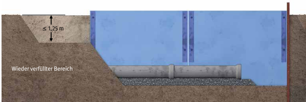
Abb. 111 Sicherung der Stirnseite des Verbaus
