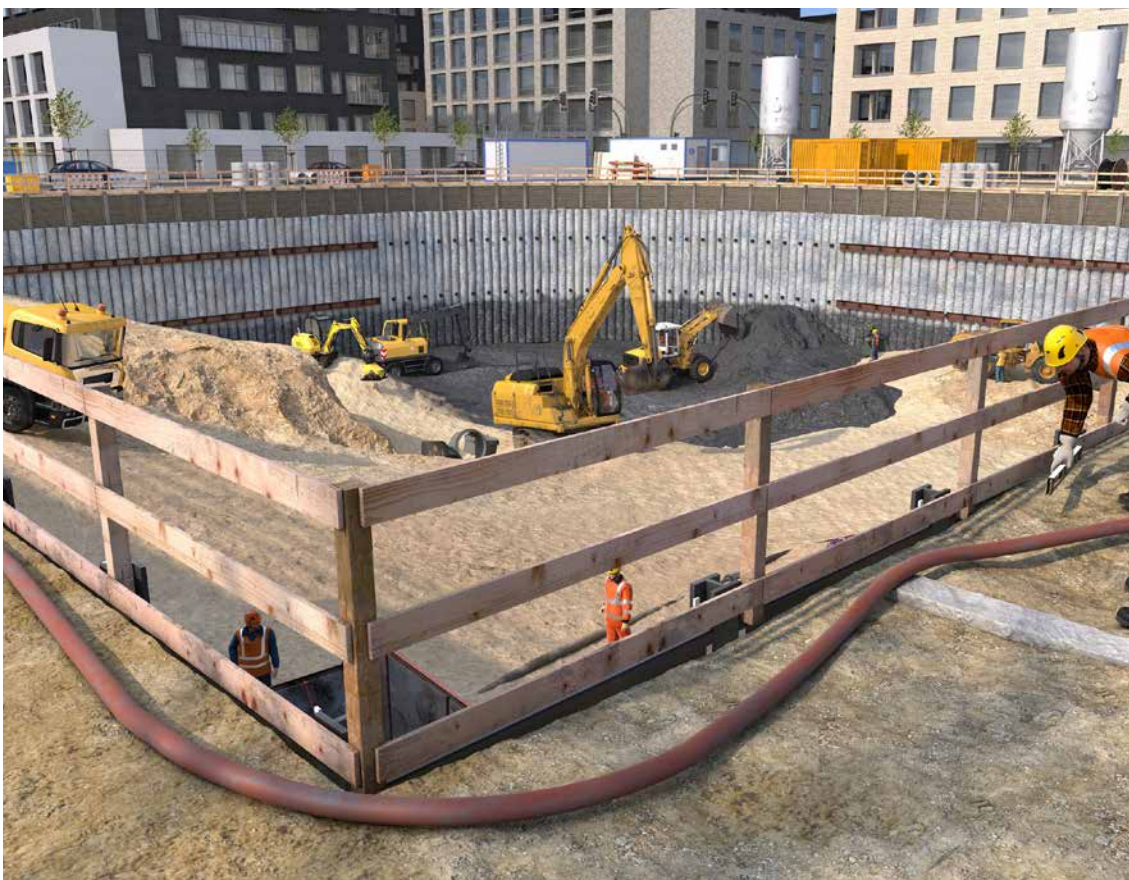
Abb. 2 Dreiteiliger Seitenschutz als Absturzsicherung an Baugruben
