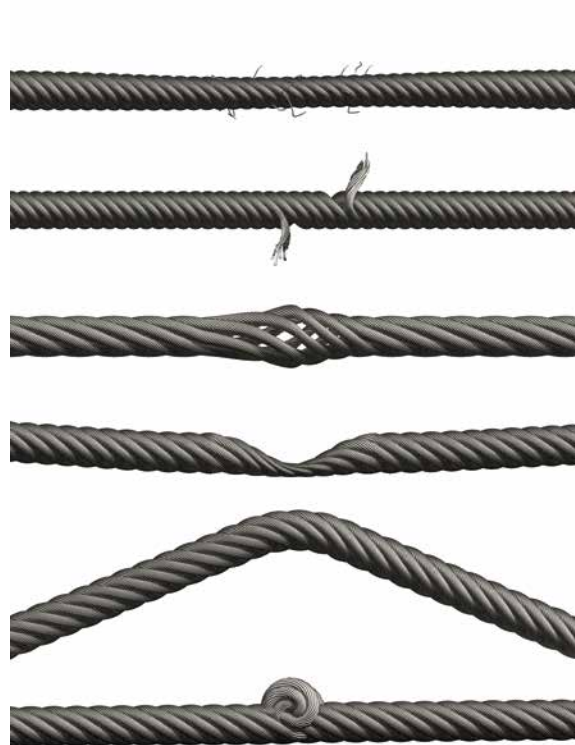
Abb. 59 Beispiele für Ablege Kriterien von Drahtseilen
