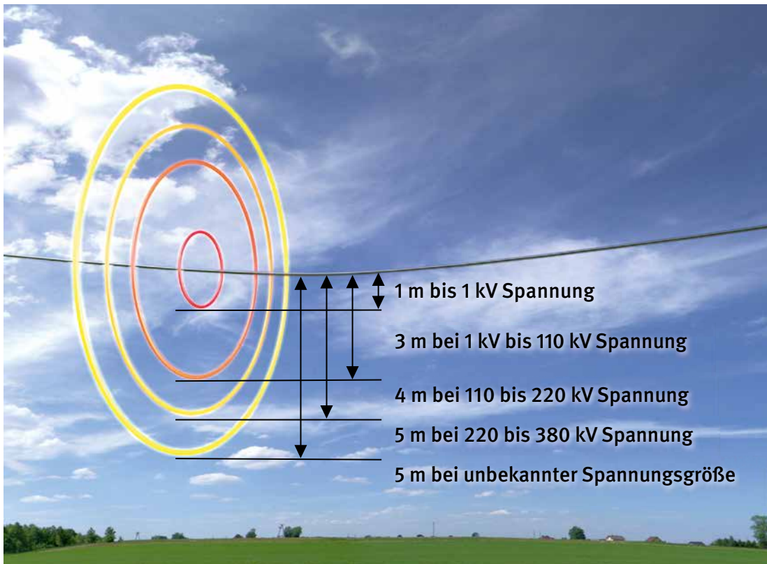
Abb. 20 Schutzabstände zu Freileitungen
