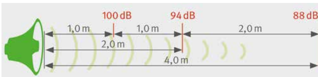
Abb. 43 Schallpegelabnahme durch Vergrößerung der Entfernung von der Lärmquelle
