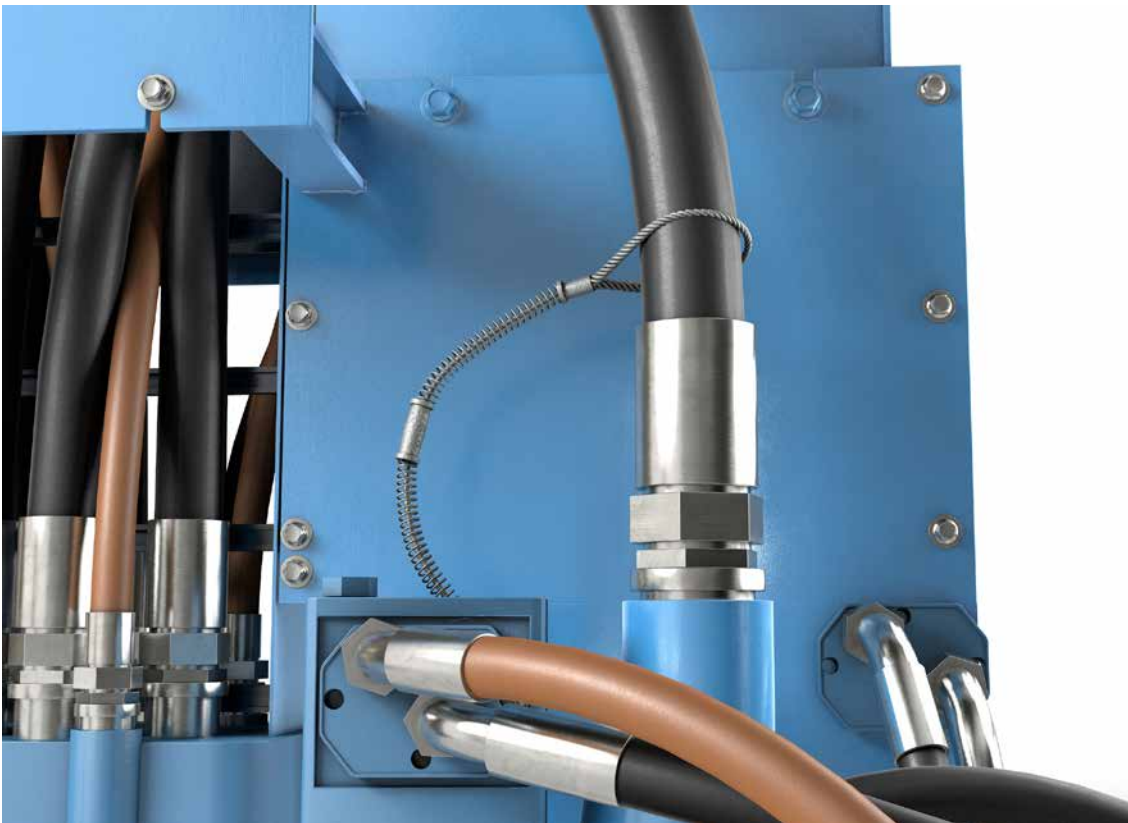
Abb. 129 Fangeinrichtung
