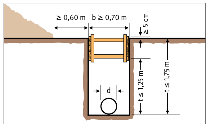
Abb. 110 Sicherung von Gräben bis 1,75 m Tiefe
