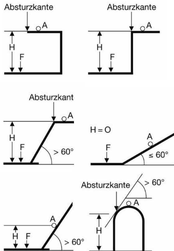
Abb. 3 „h“ = senkrechter Höhenunterschied zwischen Arbeitsplatz „A“ bzw. der Absturzkante und der Auftreffstelle „F“
