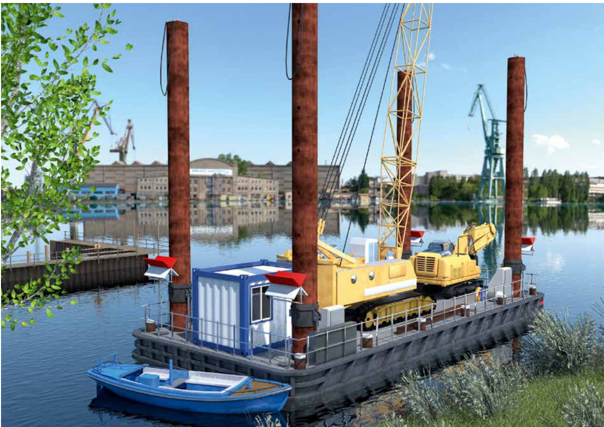
Abb. 144 Schwimmendes Gerät mit Seilbagger und Hydraulikbagger an Bord
