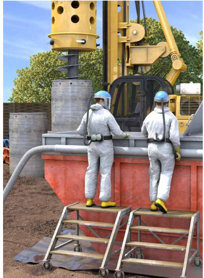
Abb. 18 Persönliche Schutzausrüstungen bei Arbeiten in kontaminierten Bereichen
