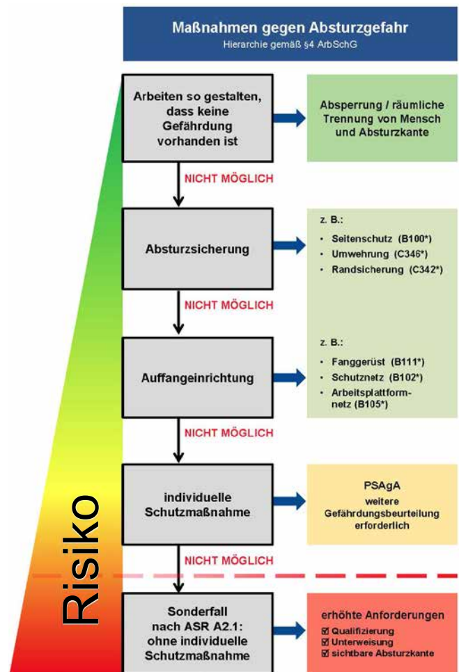
Abb. 4 Maßnahmen gegen Gefährdungen durch Absturz gemäß Arbeitsschutzgesetz
