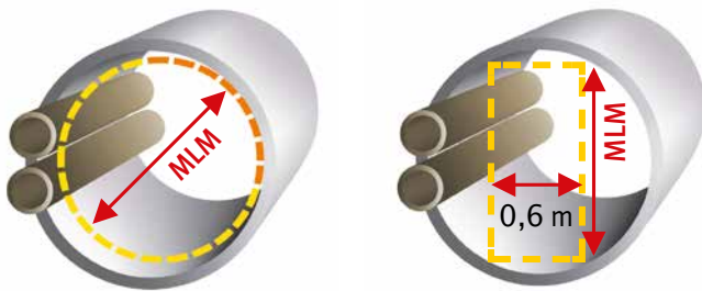
Abb. 137 Ermittlung der Mindestlichtmaße
