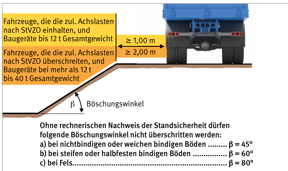
Abb. 79 Mindestabstände zwischen Fahrzeugen bzw. Baugeräten und Böschungskanten zur Wahrung der Standsicherheit
