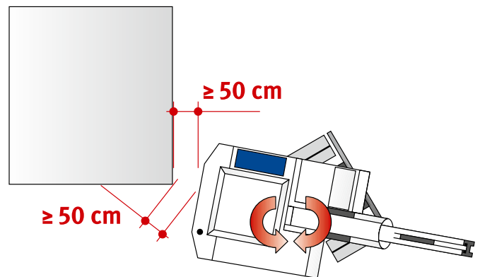
Abb. 128 Mindestabstände
